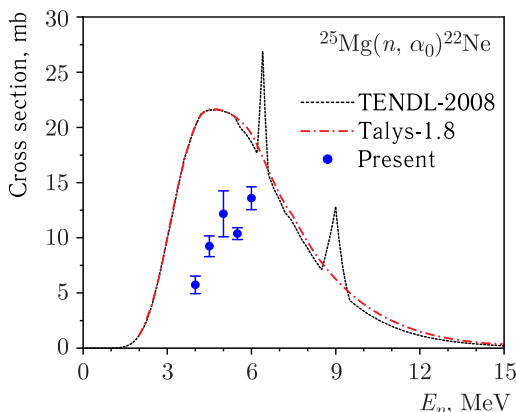
Сечение реакции ^{25}\text{Mg}(n, \alpha_0)^{22}\text{Ne} в сравнении с имеющимися экспериментальными данными, библиотеками и расчетами по Talys-1.8
