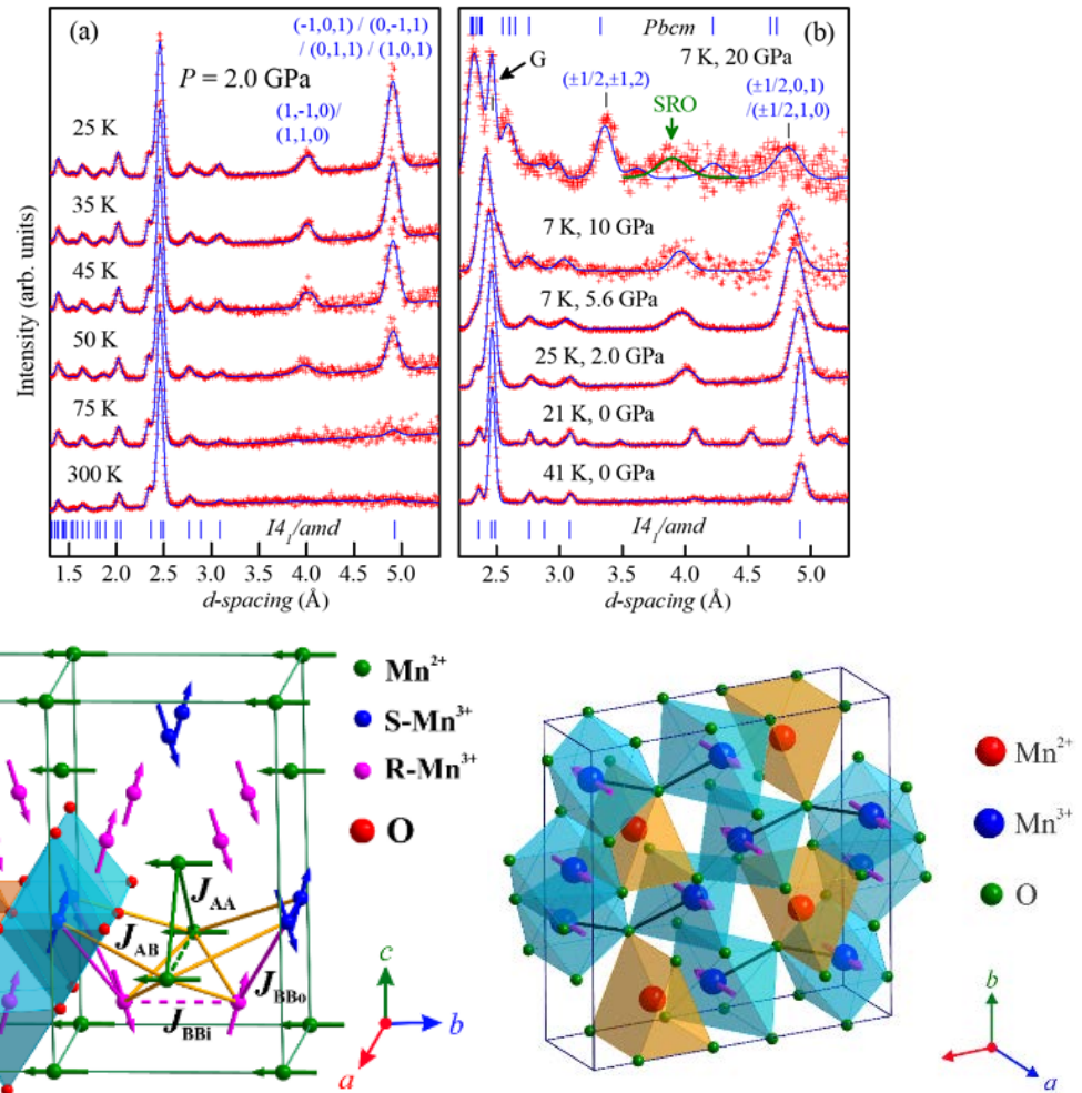
Рис. 26. Индуцированный давлением колоссальный рост температуры магнитного упорядочения в геометрически фрустрированном оксиде Mn_3O_4
