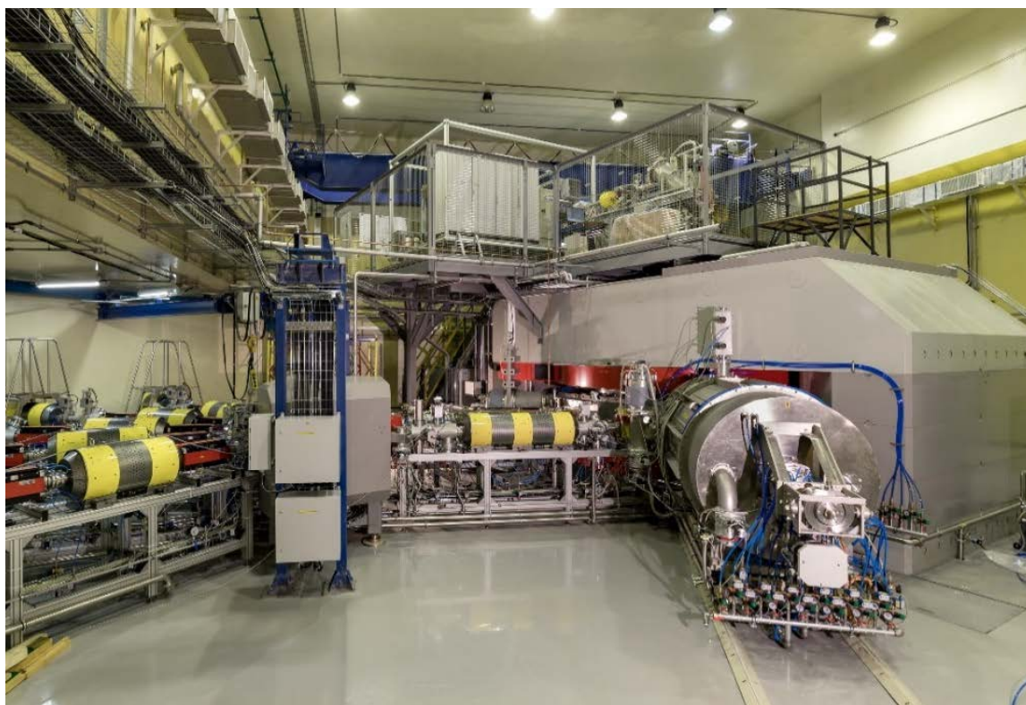
Рис. 20. Циклотрон ДЦ-280 Фабрики СТЭ
