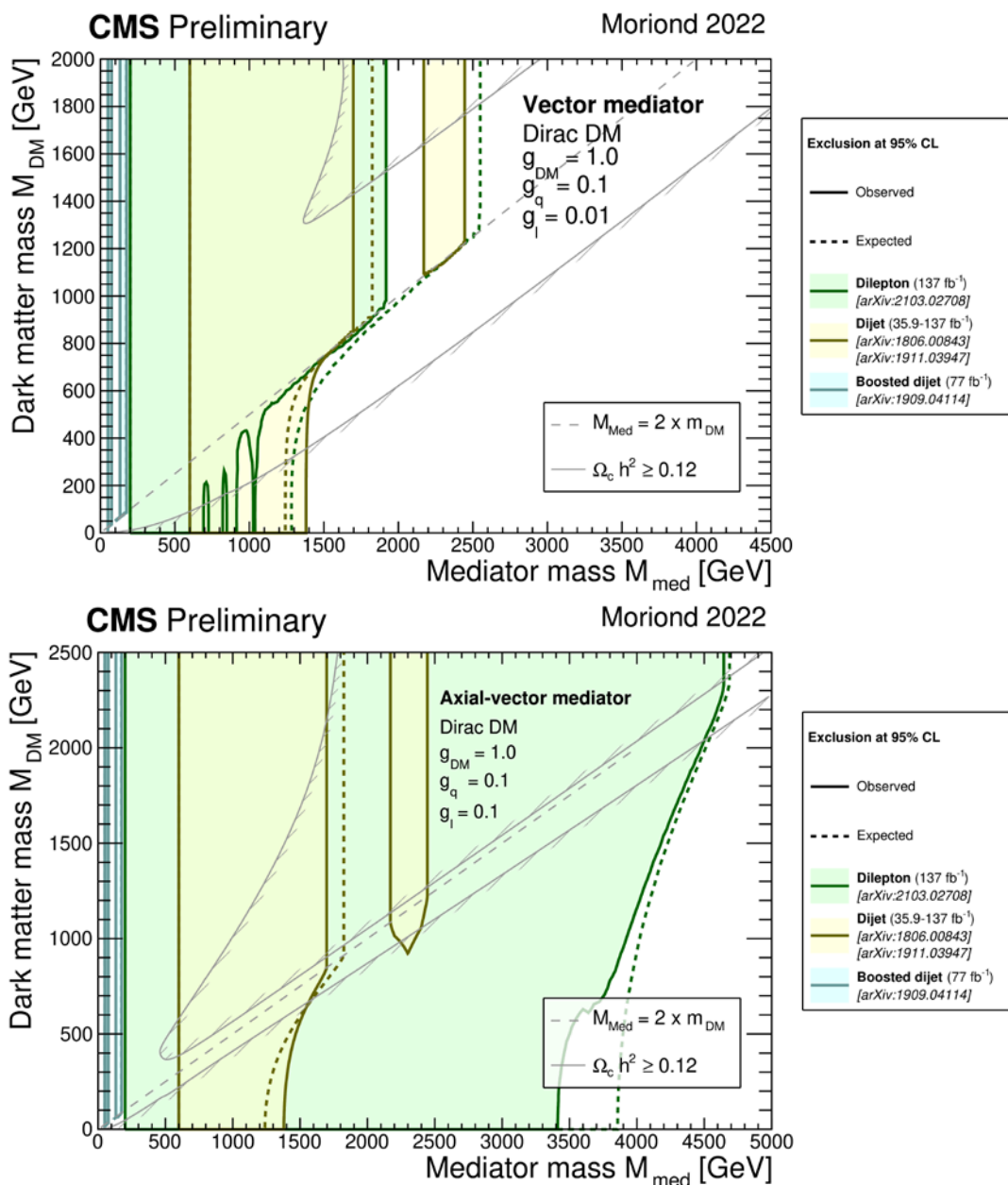
Рис. 16. В объединенном канале рождения пары струй и пары лептонов в событиях, зарегистрированных в эксперименте CMS на LHC, определены пределы (95% С.Л.) на массы частиц-кандидатов на роль частиц темной материи m_{DM} и частицы-переносчика взаимодействия с темным сектором M_{med} . Закрашенная область соответствует закрытым значениям масс для векторного (вверху) и псевдовекторного (внизу) переносчика
