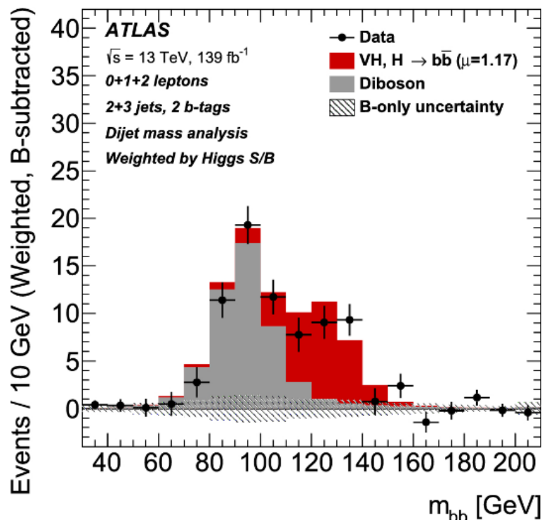
Рис. 15. Полученное в pp -взаимодействиях при энергии 13 ТэВ в эксперименте ATLAS распределение по инвариантной массе двух b -струй в процессах ассоциированного рождения бозона Хиггса с W - и Z -бозонами и его распадом на два b -кварка. Вычтен вклад всех фоновых процессов, за исключением двухбозонных – WZ и ZZ
