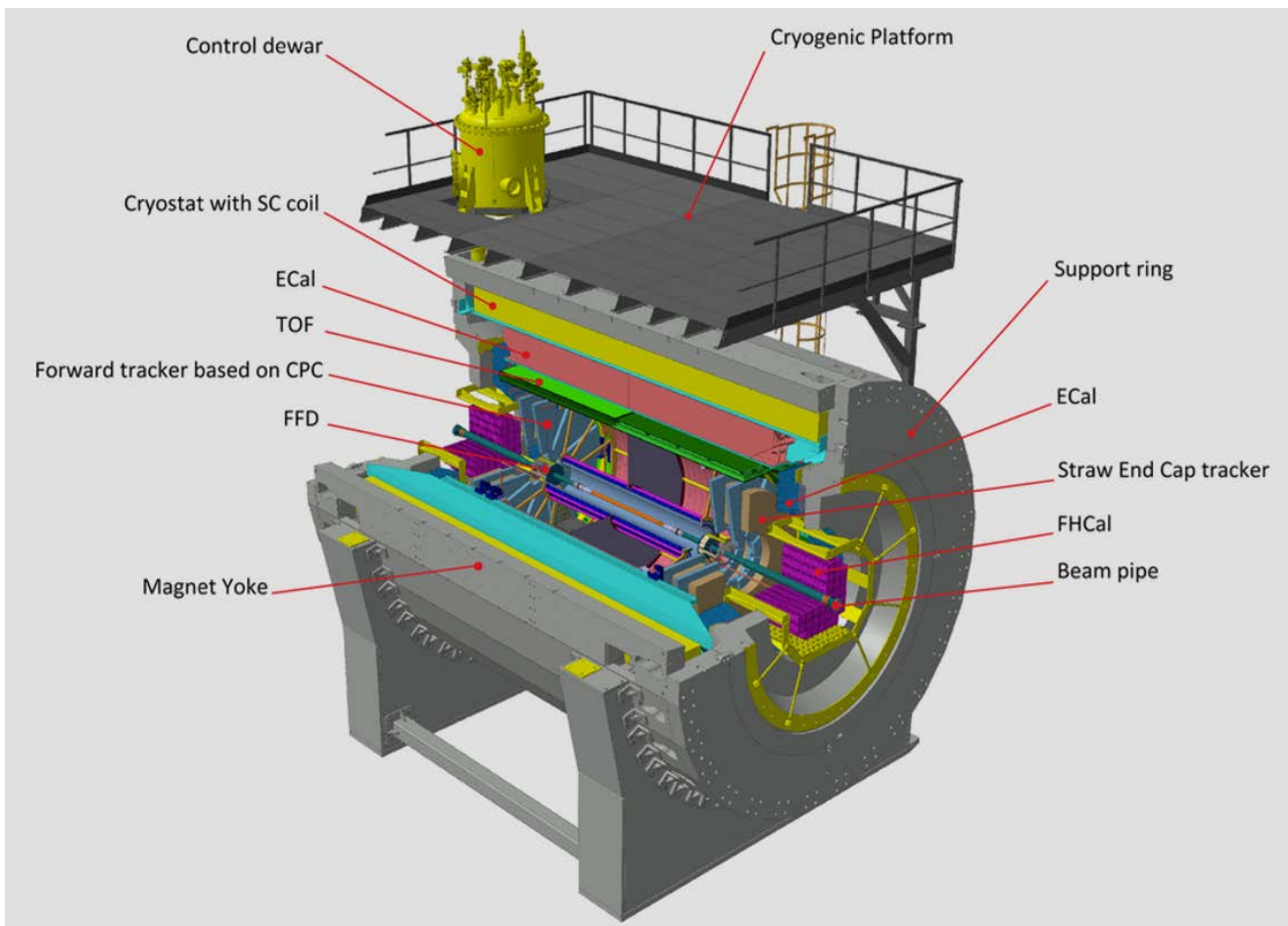
Рис. 4. Общая схема многоцелевого детектора (MPD)
