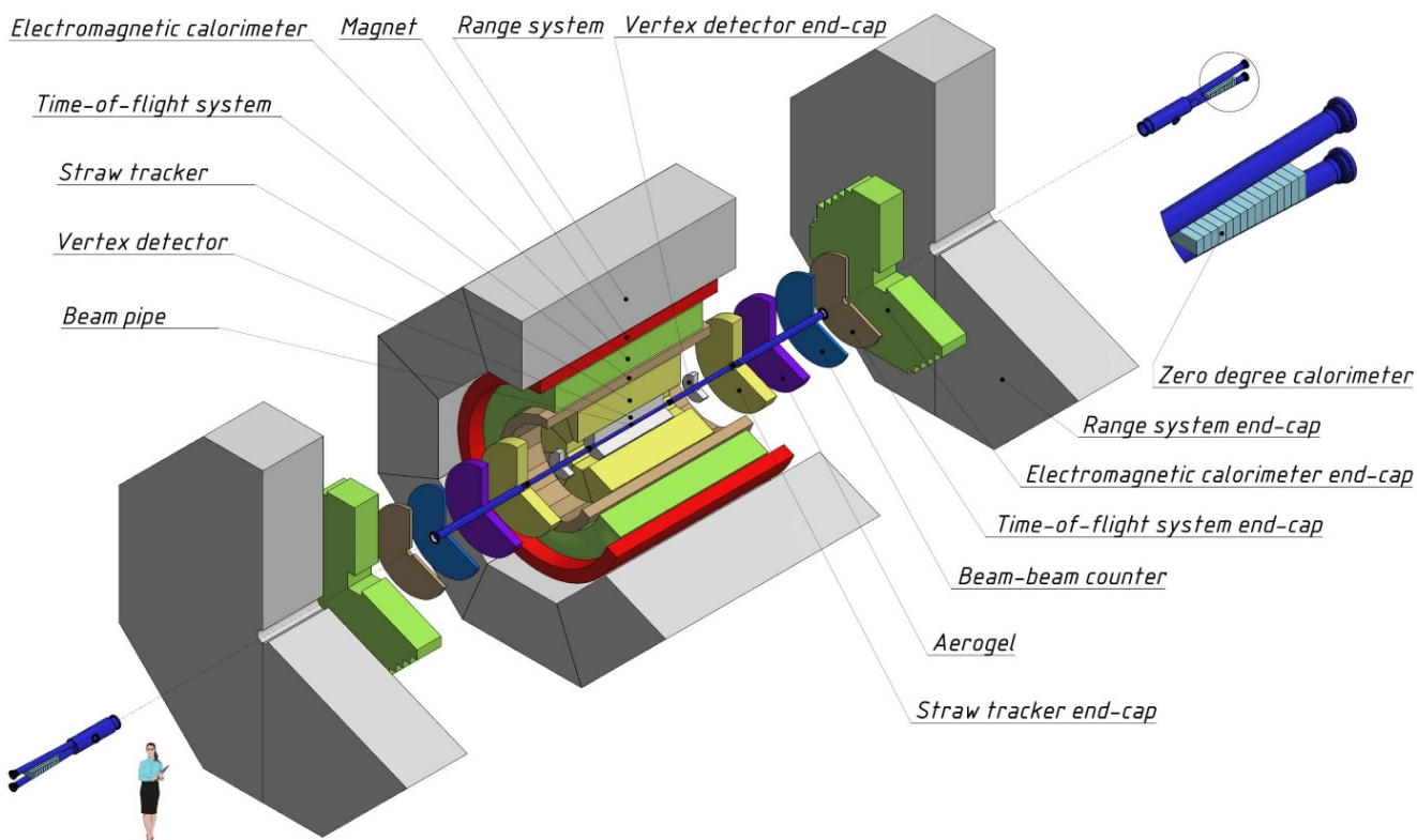
Рис. 5. Общая схема детектора спиновой физики (SPD)
