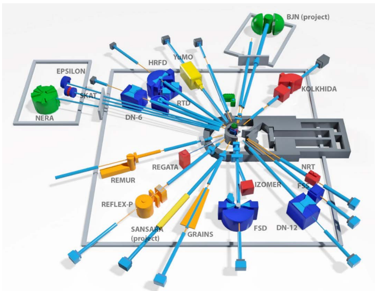
Рис. 7. Комплекс спектрометров реактора ИБР-2
