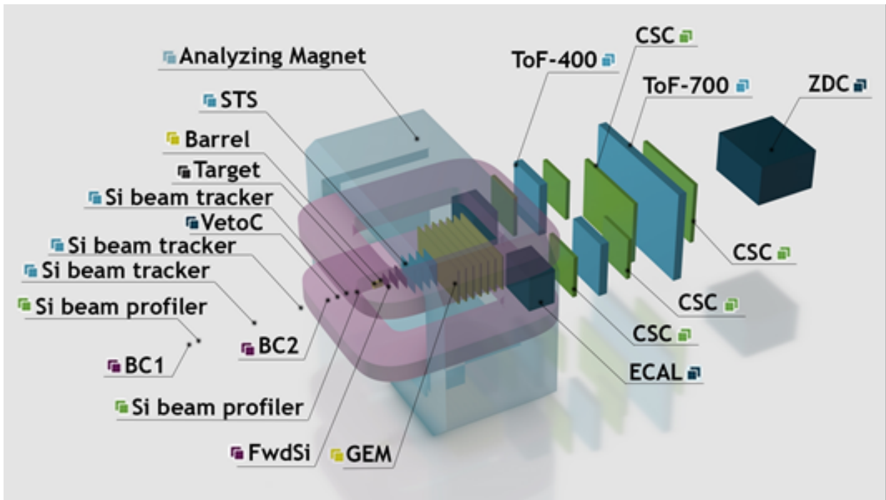
Рис. 3. Полная конфигурация детекторов ВМ@N для реализации программы исследований в пучках тяжелых ионов
