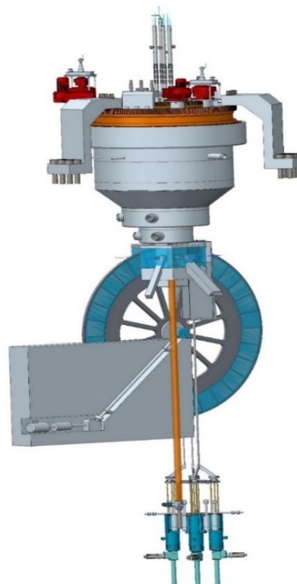
Рис. 8. Вариант нового реактора НЕПТУН
