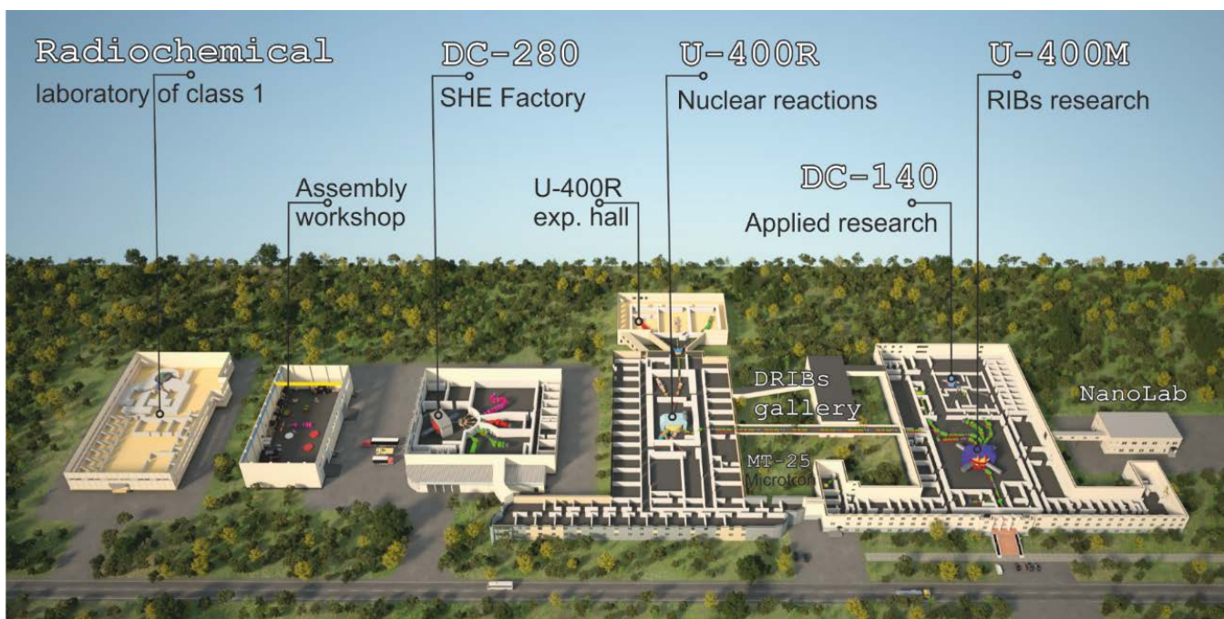
Рис. 6. План Лаборатории ядерных реакций с учетом объектов инфраструктуры, планируемых к строительству в 2024-2030 гг.
