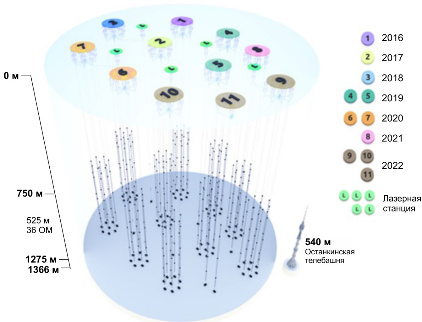
Рис. 10. Статус развертывания телескопа по состоянию на конец 2022 года. Установка содержит 2916 оптических модулей и семь лазерных калибровочных источников света на пяти станциях
