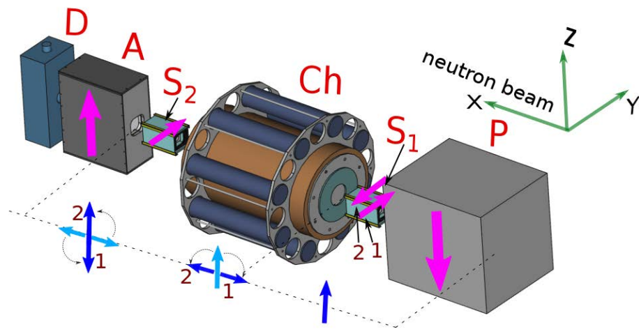
Рис. 23. Схема эксперимента для измерения T-нечетных эффектов в делении. P – SEOP поляризатор; Ch – камера деления, окруженная гамма-детекторами; A – анализатор; D – детектор нейтронов; S1, S2 – устройства управления спином. Розовые стрелки на рисунке указывают направление магнитного поля, синие стрелки – направление спина нейтрона
