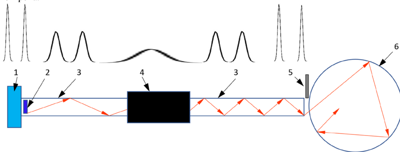
Рис. 25. Идея источника УХН для импульсного источника с использованием временной фокусировки. 1 – замедлитель, 2 – конвертер УХН, 3 – зеркальный нейтронвод, 4 – фокусирующее устройство, 5 – быстрый затвор, 6 – ловушка УХН
